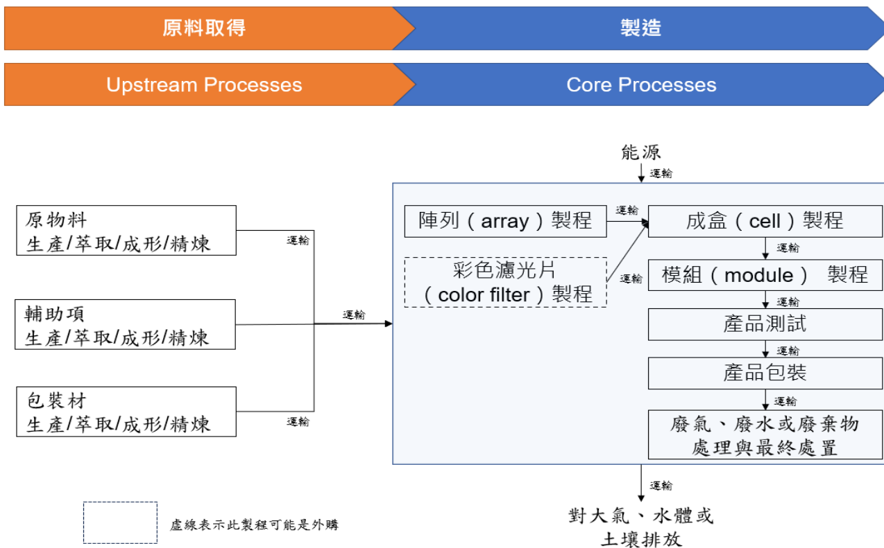
圖1、本產品類別中LCD/OLED/Micro LED顯示模組子類別的系統圖
