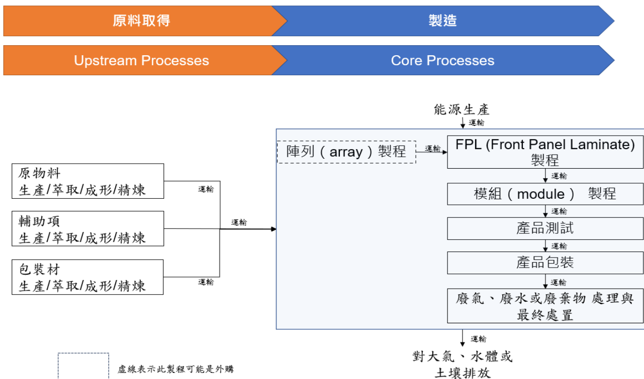
圖2、本產品類別中電子紙子類別的系統圖
